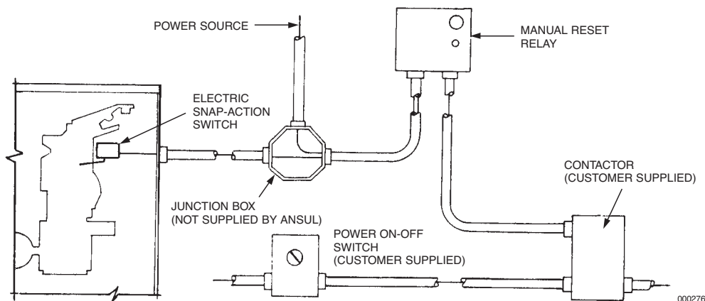
WIRING SCHEMATIC
